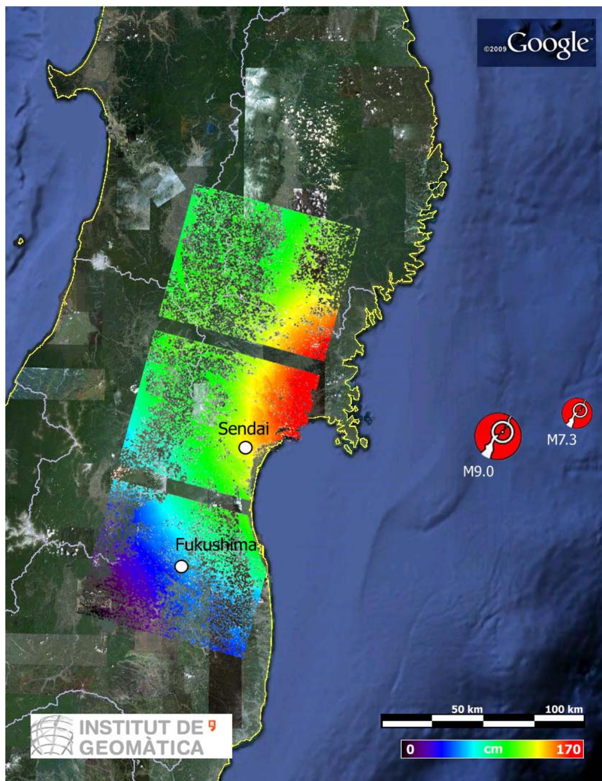
Figura 1: mapa de les deformacions co-sísmiques del terremòl de Japó (11 de març de 2011) visualitzat sobre una imatge de Google Earth. Les deformacions han estat estimades a partir de dades SAR del sensor ASAR-Envisat de l'Agència Espacial Europea. Els cercles vermells indiquen la posició de l'epicentre dels dos terremòls de magnitud superior pròxims a la zona i que han tingut lloc en el període analitzat. La imatge original està disponible a www.ideg.es .
